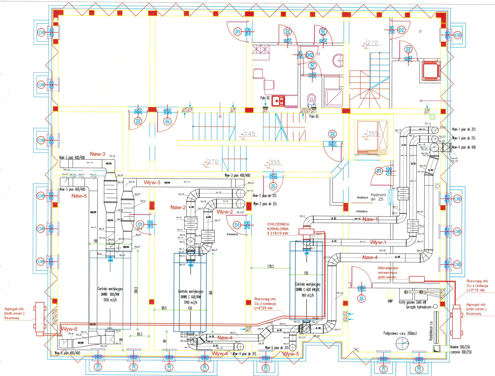
Rzut piwnic skala 1:50
